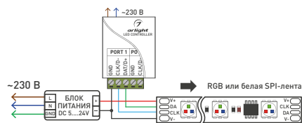
Рис. 2. Подключение светодиодной ленты или модулей с интерфейсом SPI.
