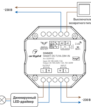
Рисунок 1. Схема подключения диммера SMART-D17-DIM
