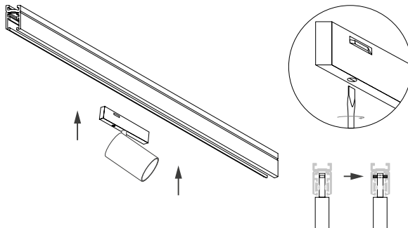
Рис. 2. Установка светильника
