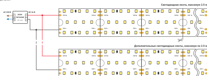
Схема 1. Параллельное подключение нескольких светодиодных лент
